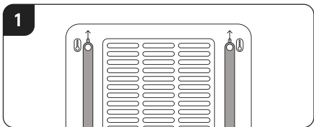
Fjern/fastgør stativet
